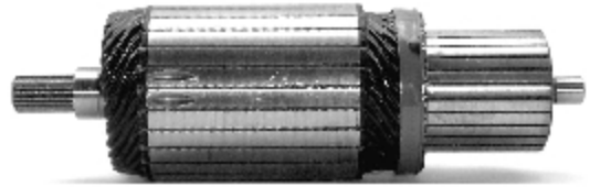
IM 3170 12 V 2.0 Kw Replacing: 028200-6860, 28160-54380 Servicing: 228000-2120, 228000-2680, 228000-2690, 228000-2700, 228000-2980, 228000-3840, 228000-3850, ... Slots:27 Teeth:21 O.D. 50,45 L. 159,7
