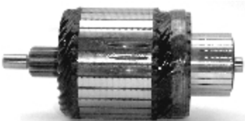
IM 3165 12 V 1.6 Kw Servicing: 228000-9900, 228000-9901, 228000-9902, 28100-0H060, 28100-0H061, 28100-28041, 28100-28041, ... Slots:29 Teeth:9 O.D. 50,55 L. 108,7
