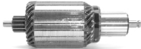
IM 3141 24 V 5,5 Kw Replacing: 1658732, 6033AD5148 Servicing: 0001241001, 0001241003, 0001241004, 0001241005, 0001241006, 0001241007, 0001241014, ... Slots:23 Teeth:13 O.D.60,0 L. 174,5
