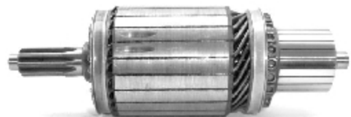
IM 3133 24 V 4.5 Kw Replacing: 0-24100-0030 Servicing: 0-24000-3030 Slots:23 Teeth:9 O.D.60,00 L. 186,5
