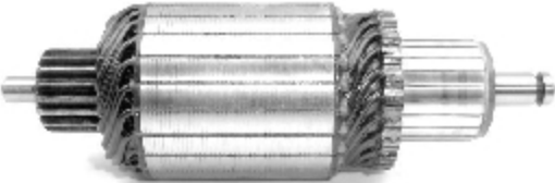
IM 2133 24 V Replacing: 039038630, 049911311C, 138254, 2004012023, 9003334024 Servicing: 0001219001, 0001219002, 0001219003, 0001219004, 0001219005, 0001219006, 0001219007, ... Slots:23 Teeth:18 O.D.50,0 L.158,0
