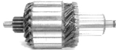
IM 2137 12 V Replacing: 233698, 6033AD0446, 6033AD1061, 6033AD1104 Servicing: 0001223013, 0001223014 Slots:19 Teeth:14 O.D.58,0 L.140,0
