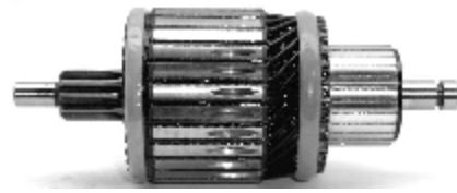
IM 3146 24 V 1.6Kw Replacing: 1004011079 Servicing: 0001111003, 0001111004, 0001111005 Slots:28 Teeth:11 O.D.55,0 L. 138,5
