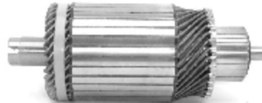
IM 307 12 V Slots: 33 O.D.74,5 L. 194,0
