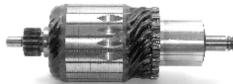
IM 3163 12 V 1.8 Kw Start&Stop Replacing: 235870 Servicing: 458414, ESW20ER121 Slots: 19 Teeth: 14 O.D. 49,7 L. 145,5
