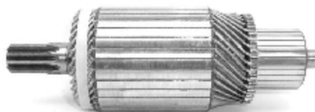
IM 3034 12 V Slots: 33 Teeth: 10 O.D. 65,0 L. 196,5
