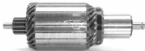
IM 3141A 24 V 5,5 Kw - WITH BEARING Replacing: 1658732, 237748, 6033AD5148 Servicing: 0001241001, 0001241003, 0001241004, 0001241005, 0001241006, 0001241007, 0001241014, ... Slots:23 Teeth:13 O.D.60,0 L. 174,5
