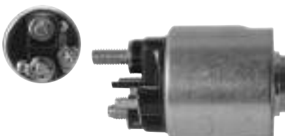
236975 Solenoid Replacing: 594414 Servicing: D6RA137, d6ra138, D6RA187, D6RA188, D6RA87 12 V, B+ M8, Kl. 50 M6, OD 54.00, OD/ cover 46.00, Total length 89.30, Height/ B+ 17.50, Width/ kl. 50 10.81, Coil bolt M8, Coil bolt 2 M8, No./ terminals 3
