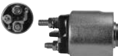
237444 Solenoid Replacing: 594444 Servicing: d6ra91 12 V, B+ M8, Kl. 50 M6, OD 53.90, Total length 89.25, Height/ B+ 30.00, Width/ kl. 50 13.00, Coil bolt M8, Coil bolt 2 22.45, No./ terminals 3
