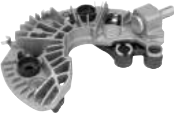
235654 Rectifier
