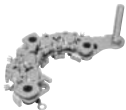
235599 Rectifier
